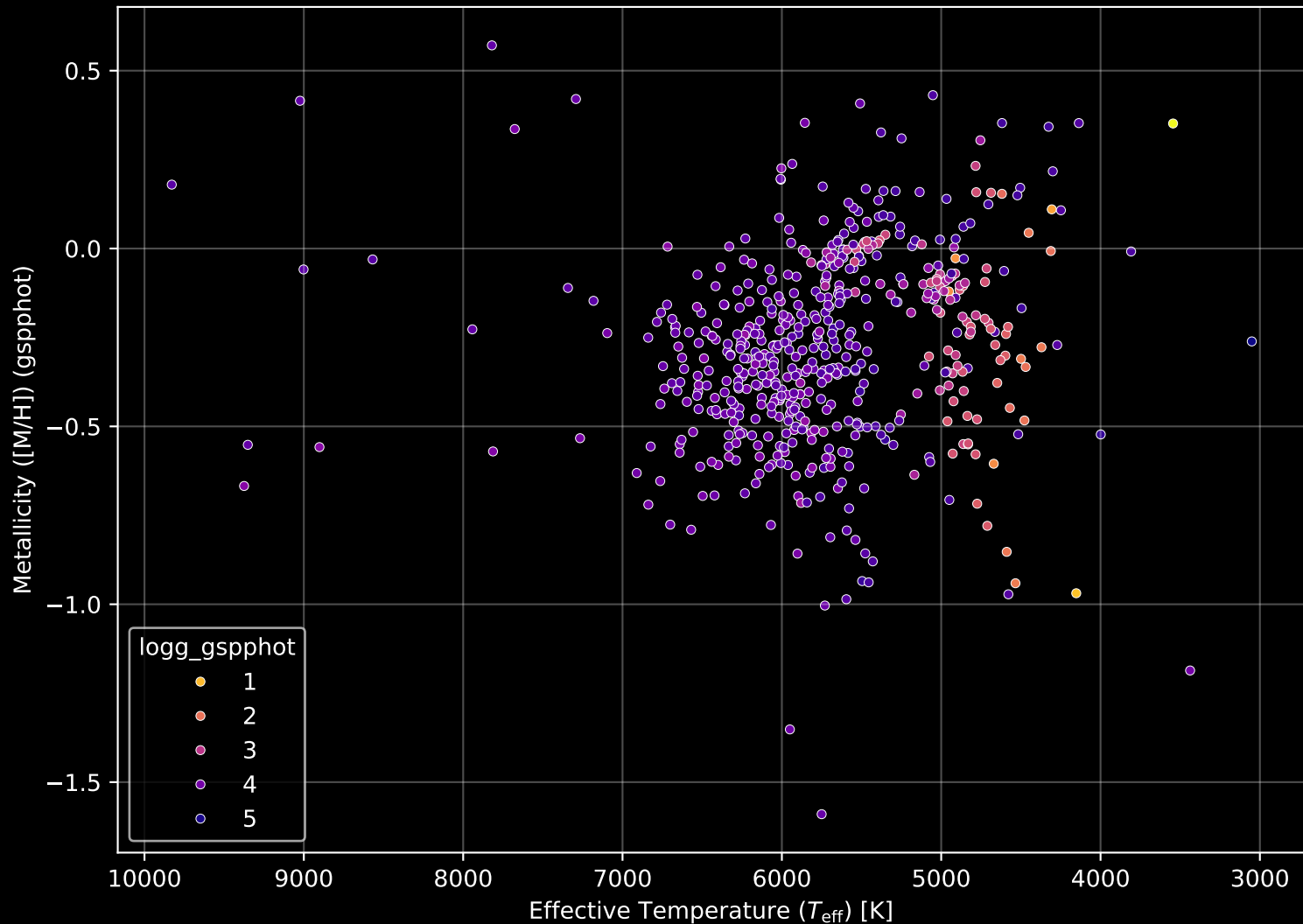
GALAH DR4 Field: [2437] Stellar Population Parameters (n= 557)
