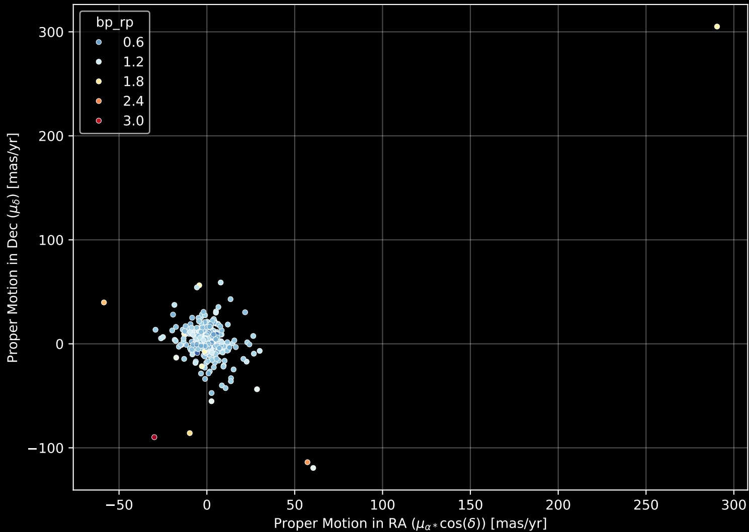
GALAH DR4 Field: [2437] Proper Motion Diagram (n= 557)
