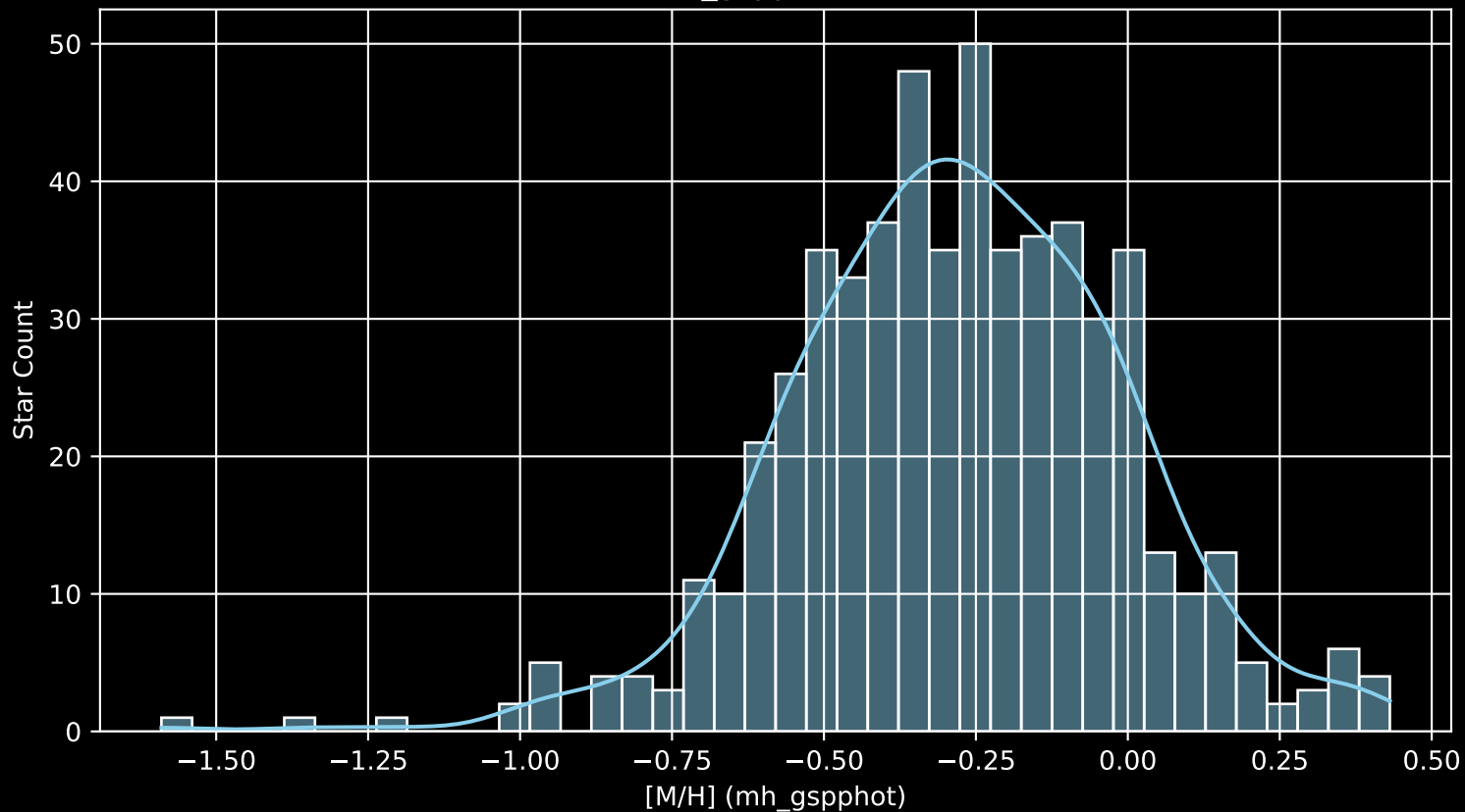
GALAH DR4 Field: [2437] [M/H] (mh_gspphot) (n= 556)
