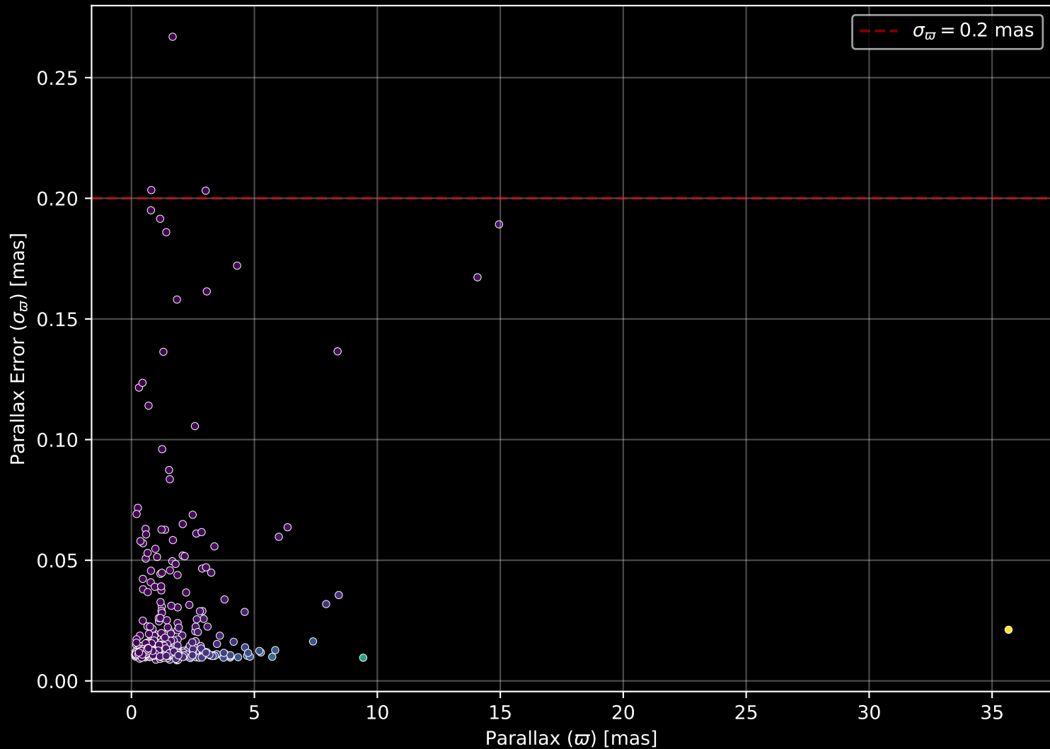
GALAH DR4 Field: [2437] Parallax Quality (n= 557)
